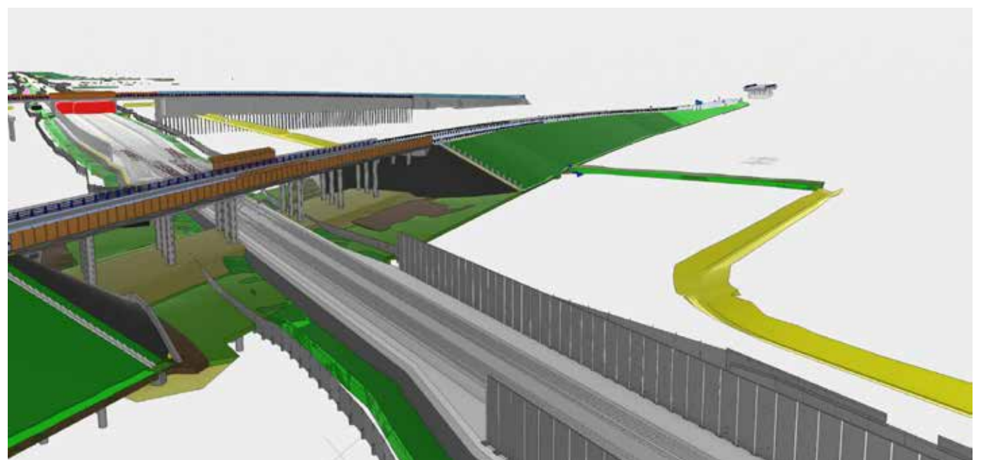
Kohila viadukt
